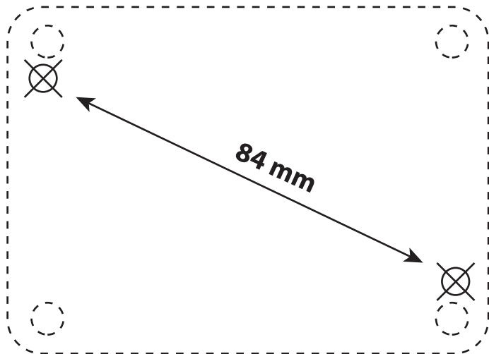
Bild 2.: Schablone für Bohrflöcher zur Befestigung des Dämmerungsschalters TS-31-2-G
