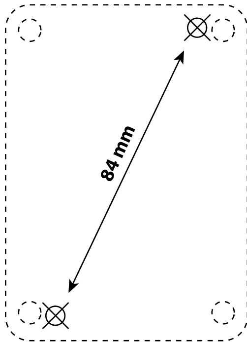
Bild 2.: Schablone für Bohrlöcher zur Befestigung des Dämmerungsschalters TS-31-2
