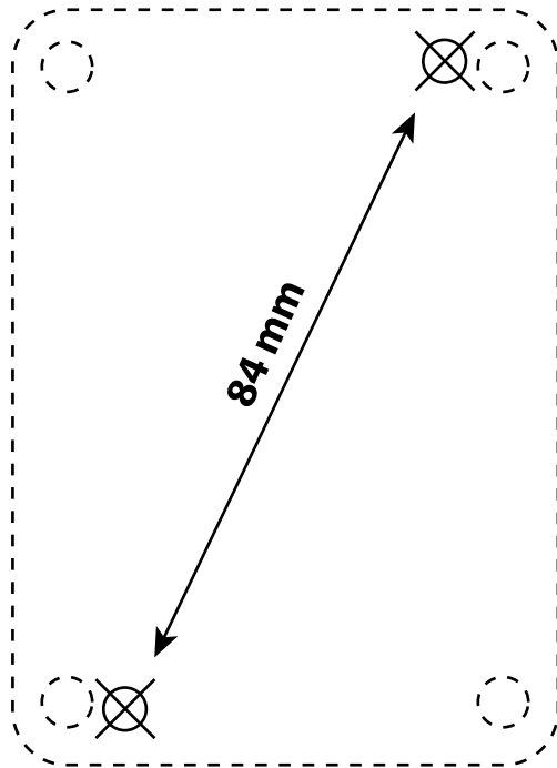
Bild 2.: Schablone für Bohrlöcher zur Befestigung des Dämmerungsschalters TS-31-1
